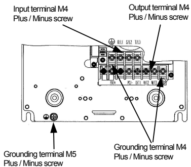
VFFS1-4007PLE-4022PLE
