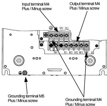
VFFS1-4037PLE-4055PLE
