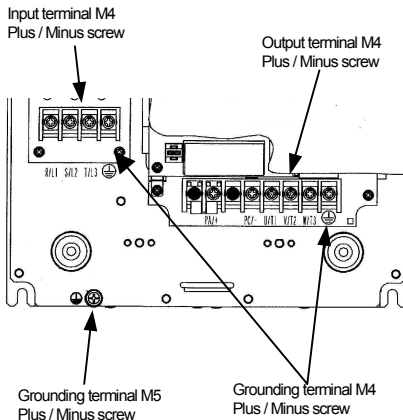
VFFS1-4037PDE-4055PDE
