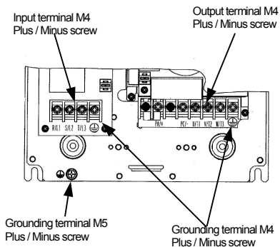
VFFS1-4007PDE-4022PDE
